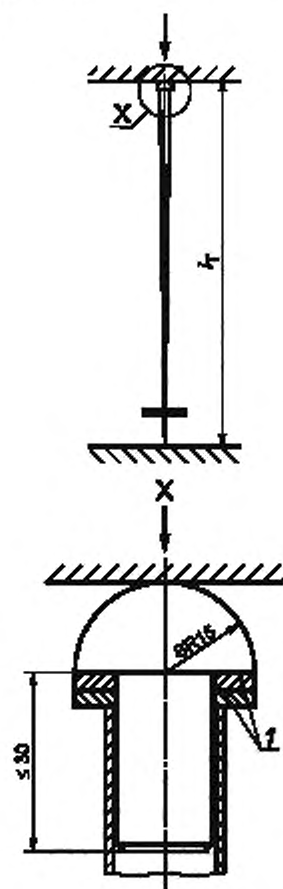
1 — компенсирующие кольца для достижения l_T
