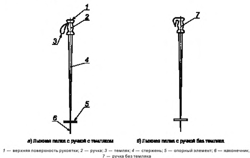
Рисунок 1 — Термины, используемые для обозначения частей лыжной палки
