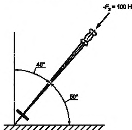
Рисунок 11 — Схема испытания на силу сцепления со льдом
