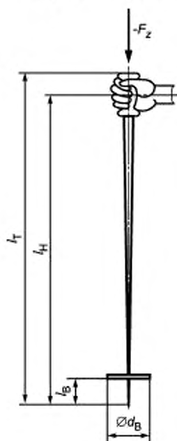
Рисунок 2 — Центр вращения и размеры
