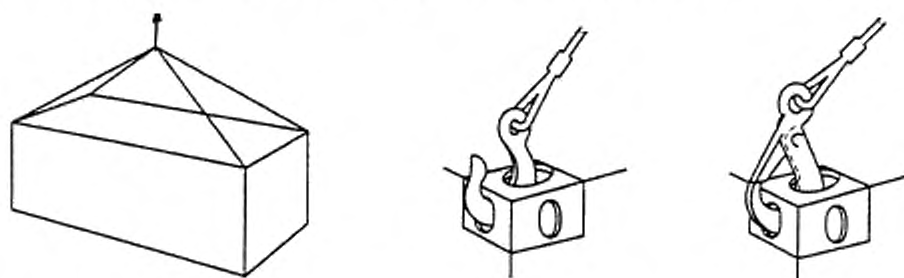
Рисунок 3 — Подъем стропами за верхние угловые фитинги
