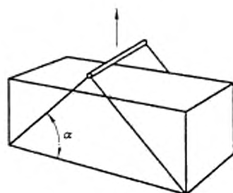
Рисунок 5 — Подъем стропами за нижние угловые фитинги
