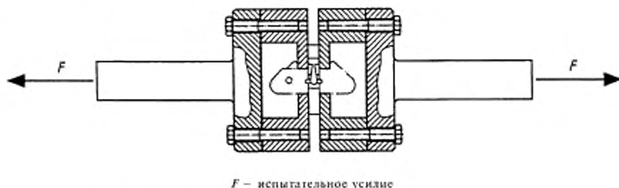
Рисунок Б.9 — Испытание стопора на растяжение
