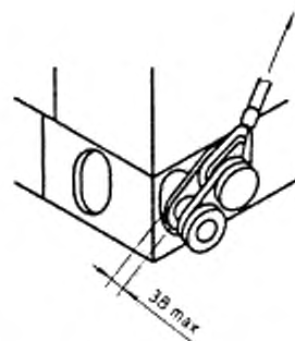
Рисунок 6 — Крепление стропа к нижнему угловому фитингу
