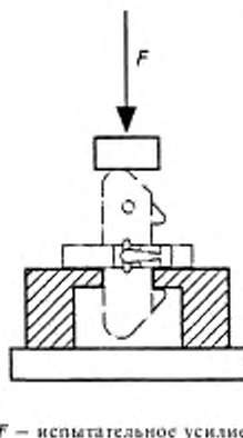
Рисунок Б.11 — Испытание конуса стопора на сжатие
