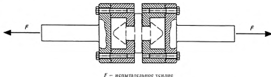
Рисунок А.10 — Испытание стопора (твистлока) на растяжение
