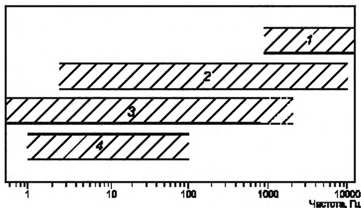
1 — пьезоэлектрические, 2 — электродинамические; 3 — гидравлические, 4 — механические
