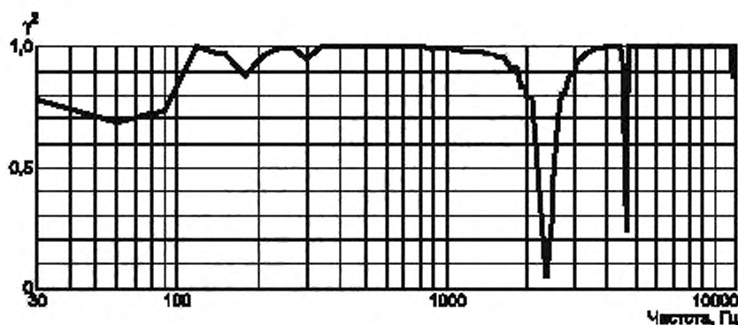
Рисунок А.1 — Типичный график функции когерентности
