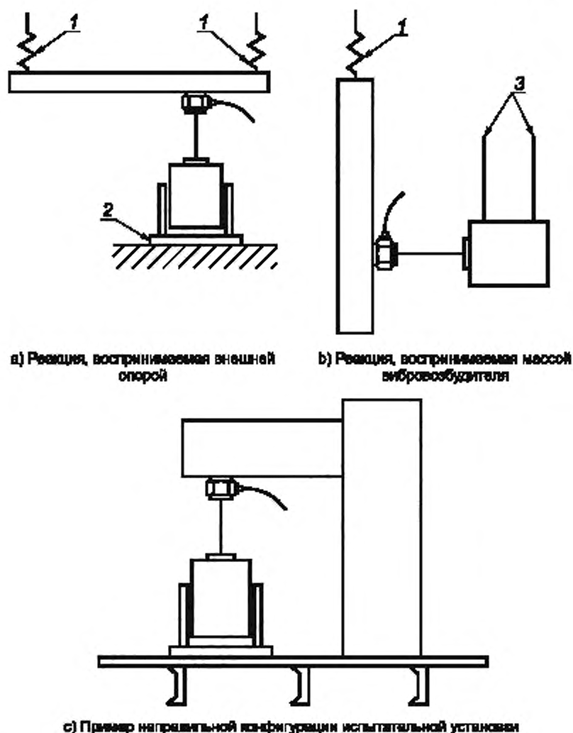
1 — подвес испытуемой конструкции; 2 — опора вибровозбудителя; 3 — подвес вибровозбудителя
