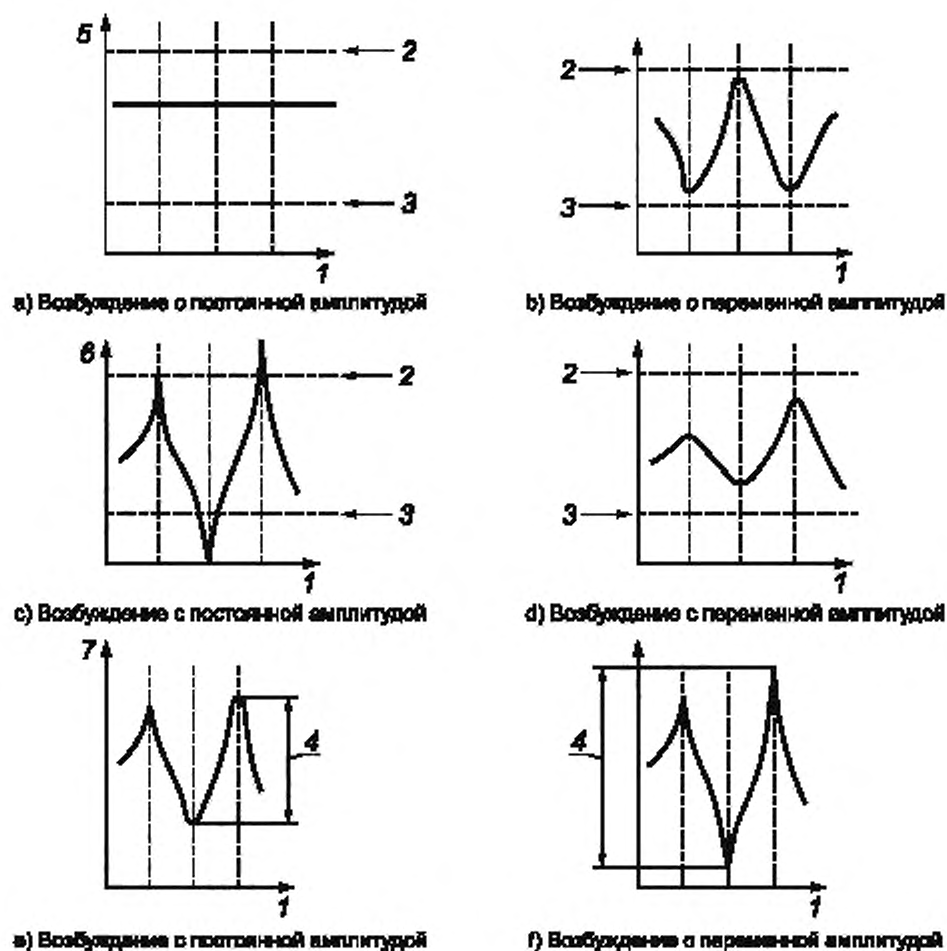
1 — частота; 2 — максимальный уровень возбуждения; 3 — шумовой порог; 4 — достижимый динамический диапазон; 5 — истинное значение амплитуды (спектральной плотности мощности) силы; 6 — истинное значение амплитуды (спектральной плотности мощности) ускорения; 7 — результат измерений частотной характеристики
