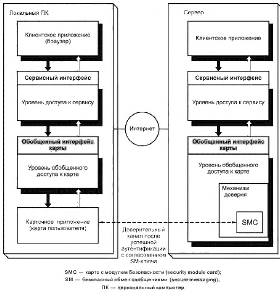
Рисунок А.10 — Распределенная реализация, использующая механизм доверия
