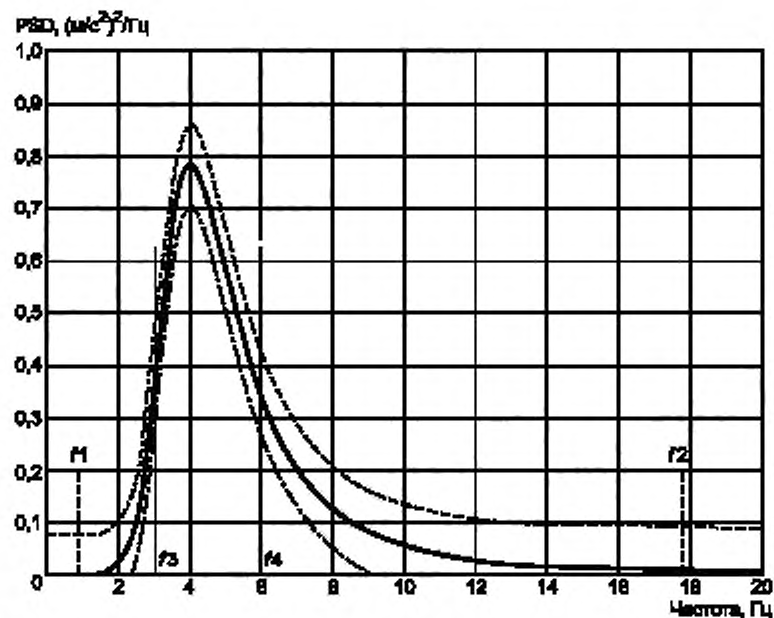
Рисунок 10 — PSD для входного спектрального класса EM 9 (погрузчик с бортовым поворотом \leq 4\,500 кг)
