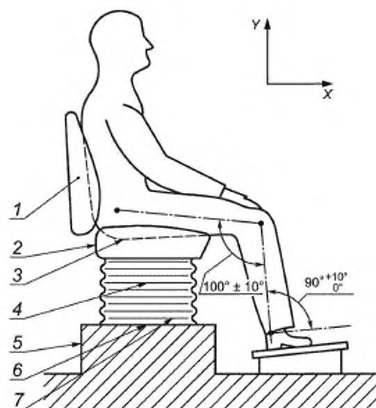
1 — спинка сиденья; 2 — подушка сиденья; 3 — диск с закрепленным акселерометром на подушке сиденья; 4 — подвеска сиденья; 5 — платформа; 6 — акселерометр, установленный на поверхности платформы; 7 — основание сиденья Должны быть приняты меры для регулировки углов в коленях и в лодыжках
