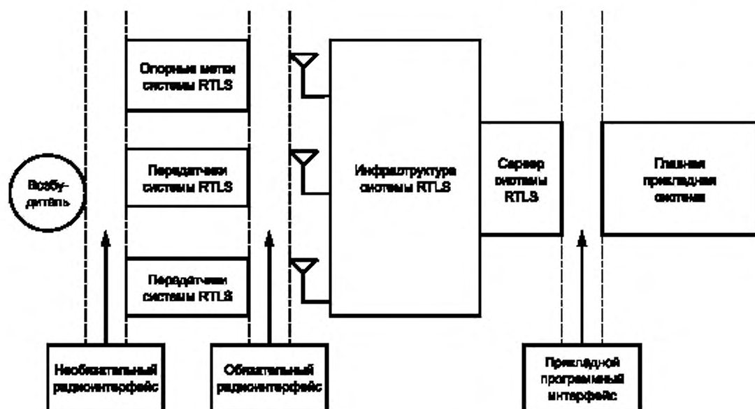
Рисунок 1 — Элементы инфраструктуры системы RTLS
