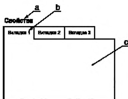
а — заголовок набора вкладок; б — заголовок вкладки; с — область отображения содержимого вкладки
