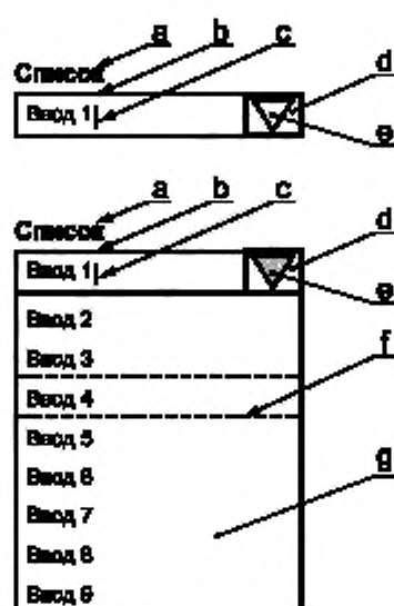
а — заголовок; б — поле ввода; с — курсор; d — кнопка списка; e — индикатор; f — курсор выбора; g — список
