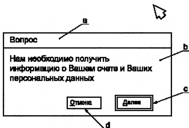
а — заголовок; б — информация; в — нажимаемая кнопка с действием по умолчанию; г — средства отмены/закрытия диалогового окна
