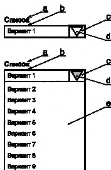
а — заголовок; б — поле данных; в — кнопка списка; г — индикатор; е — список
