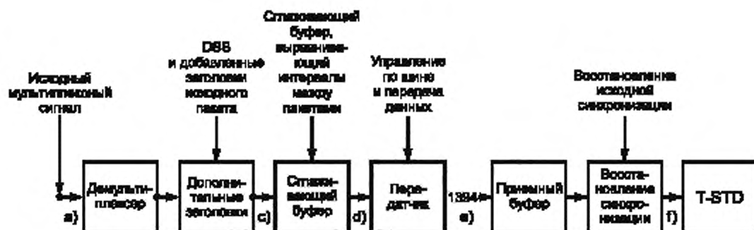
Рисунок 2 — Блок-схема обработки потока DSS
