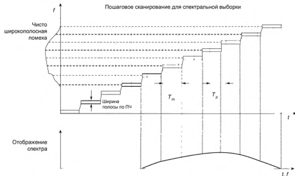
Рисунок 2 — Пример временного анализа
