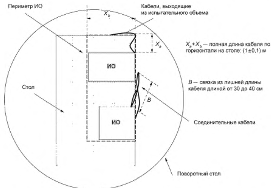
Рисунок 12 — Испытательная установка для настольного оборудования (вид сверху)
