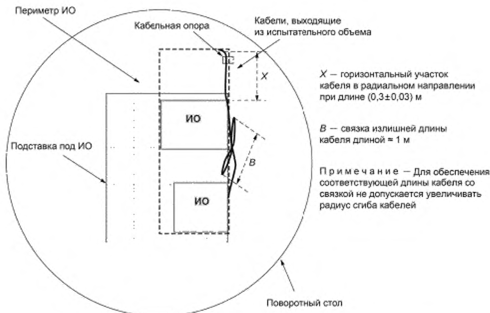
Рисунок 14 — Испытательная установка для напольного оборудования (вид сверху)
