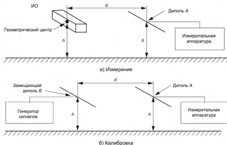
Рисунок 18 — Геометрия испытательной установки при методе замещения
