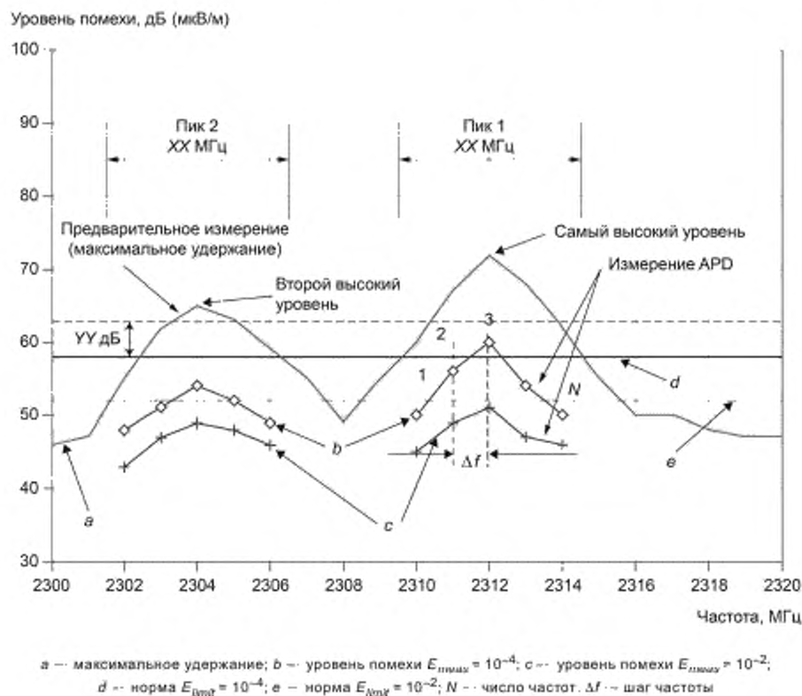
Рисунок D.1 — Пример измерения APD для флюктуирующих помех по методу 1
