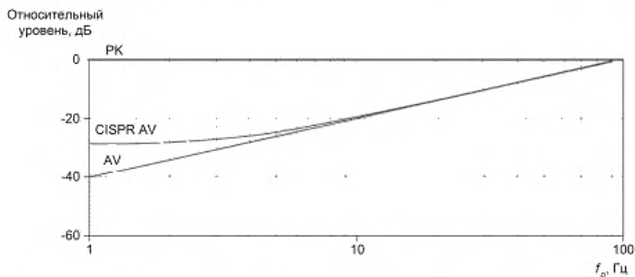
Рисунок С.1 — Весовая функция импульса 10 мс при детектировании пиковым детектором (PK) и детектором средних значений при показании в пиковых значениях (CISPR AV) и показании не в пиковых значениях (AV): постоянная времени прибора 160 мс
