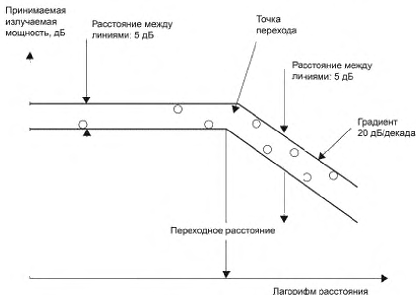
Рисунок 17 — Определение переходного расстояния
