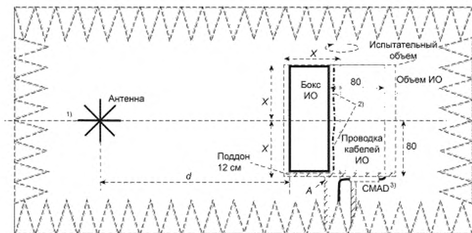
A — поворотная платформа и опора для ИО; 2X — 1,5; 2,5; 5 м; d — 3, 5 или 10 м (для испытательного расстояния 3, 5 или 10 м соответственно)
