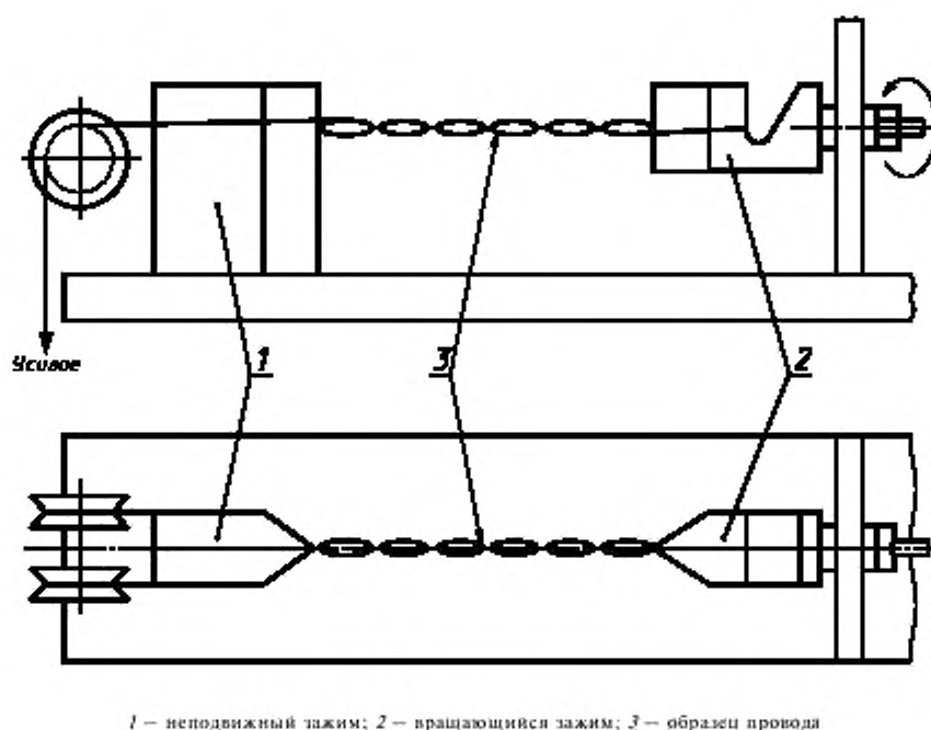
Рисунок 2 — Устройство для скручивания образца при испытании пробивным напряжением
