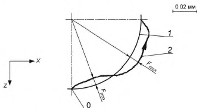
+ — центр номинальных окружностей; 0 — начальная точка; 1 — номинальная траектория, 2 — фактическая траектория. радиальное отклонение: F_{ZX, \max} = +0.008 мм, F_{ZX, \min} = -0.006 мм
