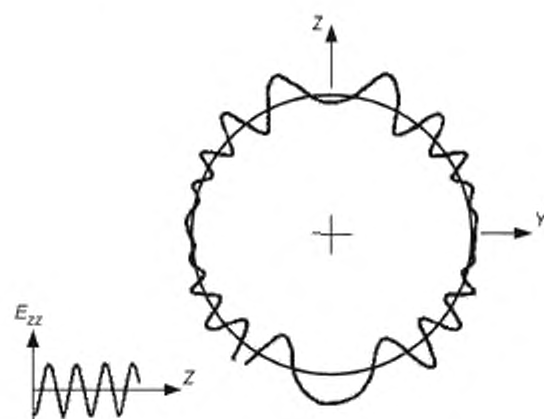
Рисунок В.3 — Влияние циклических отклонений Z
