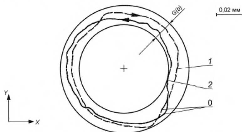
Рисунок 1 — Измерение двухнаправленного отклонения
