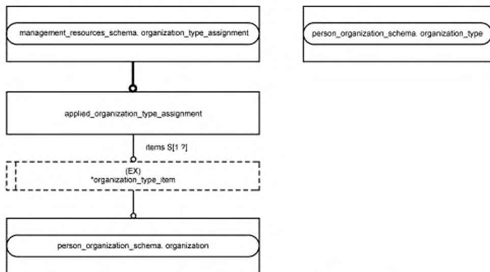
Рисунок D.2 — Представление IMM на уровне объектов в формате EXPRESS-G (диаграмма 1 из 1)
