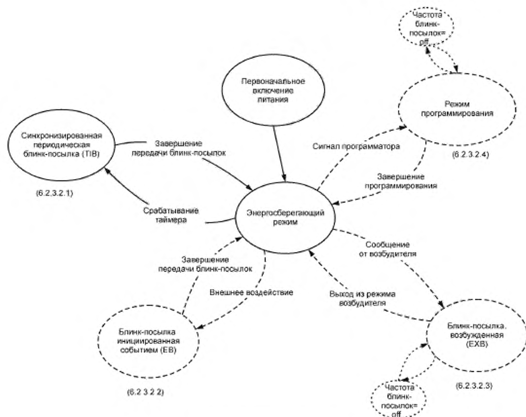
Рисунок 3 — Диаграмма состояний передатчика системы RTLS
