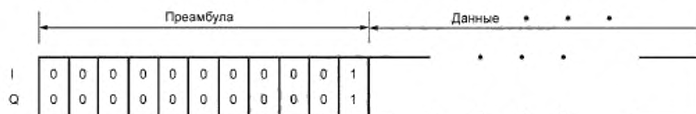
Рисунок 9 — Структура сообщения передатчика (метки) системы RTLS
