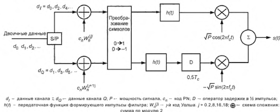
Рисунок 6 — Кодирование данных QPSK и схема расширения со смещением функции Уолша (WQPSK)
