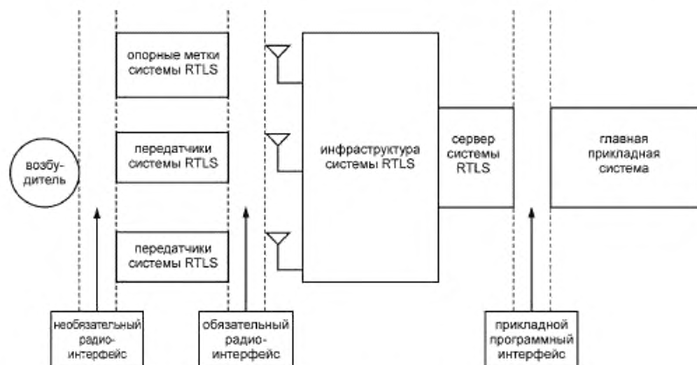
Рисунок 1 — Элементы инфраструктуры системы RTLS
