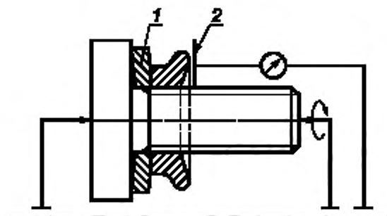
Рисунок С.22 — Измерительное устройство для проверки полного биения (перпендикулярности), установленного на рисунке 82
