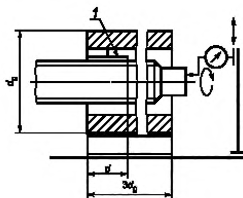
1 — трехкулачковый патрон
