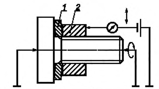
Рисунок С.21 — Измерительное устройство для проверки полного биения (перпендикулярности), установленного на рисунках 79—81
