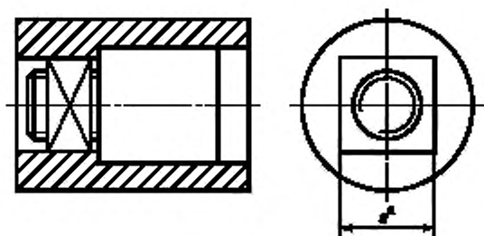
Рисунок С.18 — Калибр для проверки позиционного допуска, установленного на рисунке 75
