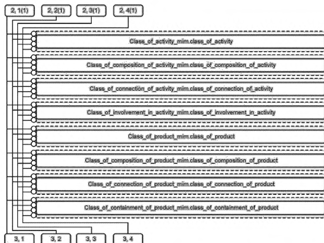
Рисунок D.4 — Представление IMM на уровне объектов в формате EXPRESS-G. Диаграмма 3 из 3
