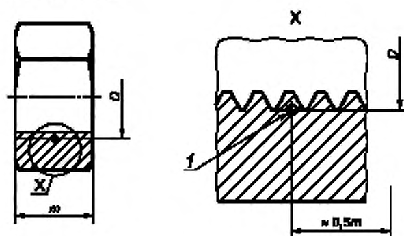
1 — Расположение точек измерения твердости
