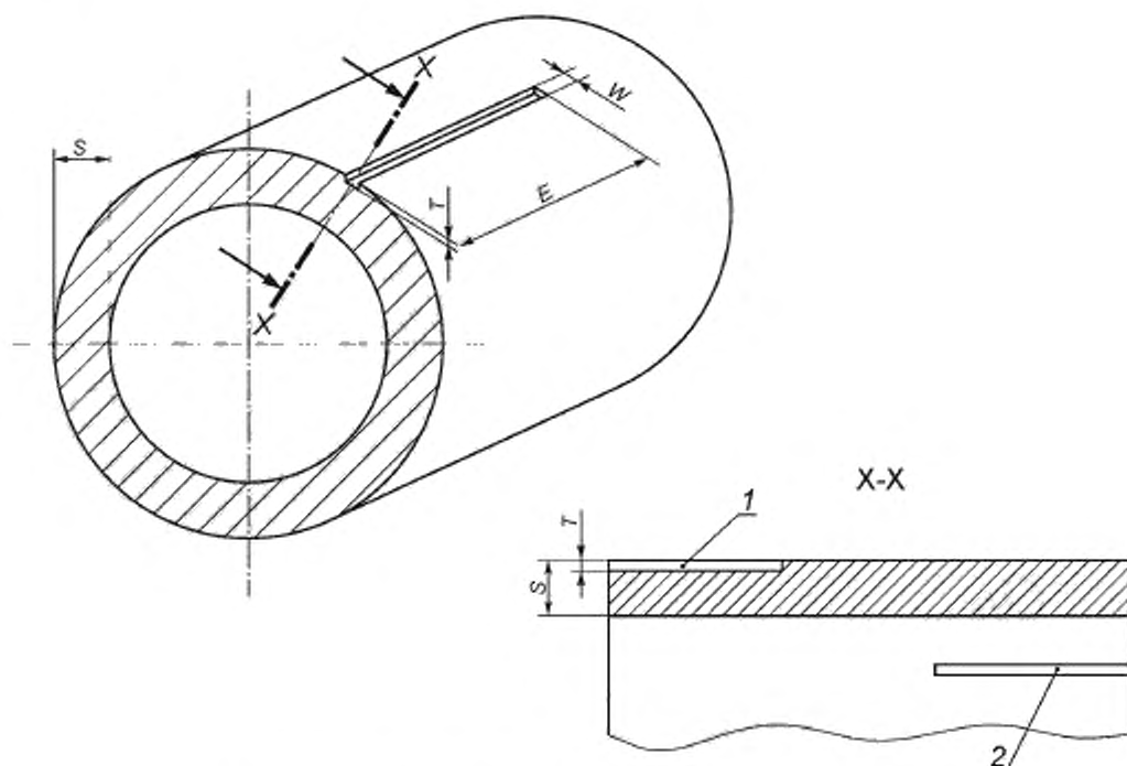
1 — наружный контрольный надрез; 2 — внутренний контрольный надрез
