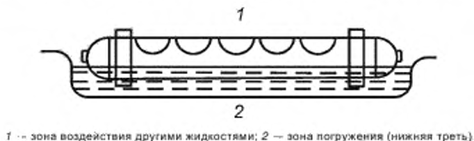
Рисунок F.2 — Расположение баллона и схема расположения зон воздействия
