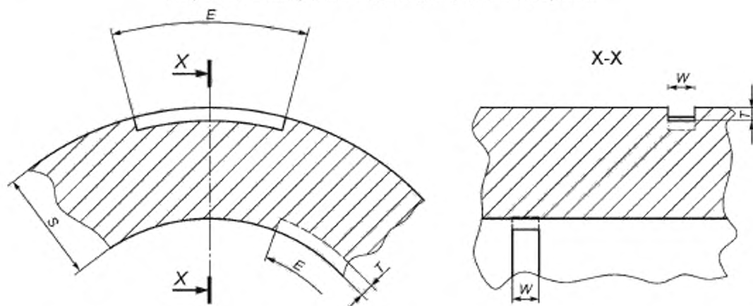
Рисунок В.1 — Контрольные надрезы для продольных дефектов
