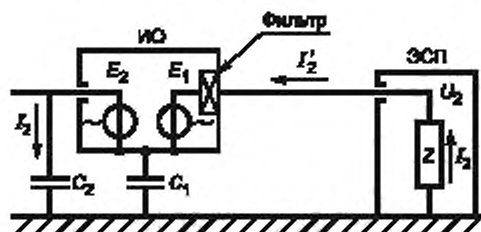
Рисунок А.3 — ИО с хорошей фильтрацией, но с неполным экранированием
