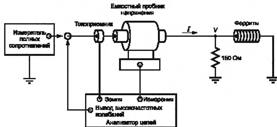
Рисунок G.4 — Основная установка для измерения полного сопротивления резистора 150 Ом и ферритов
