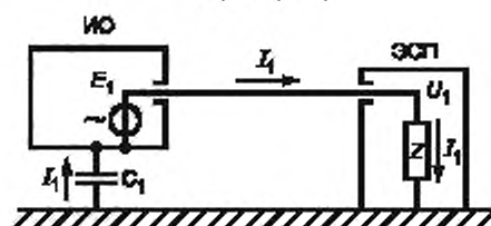
Рисунок А.5 — Подача помехи через экранированные провода
