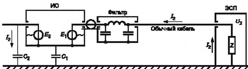
Рисунок А.6 — Подача помех через неэкранированные провода при наличии фильтра
