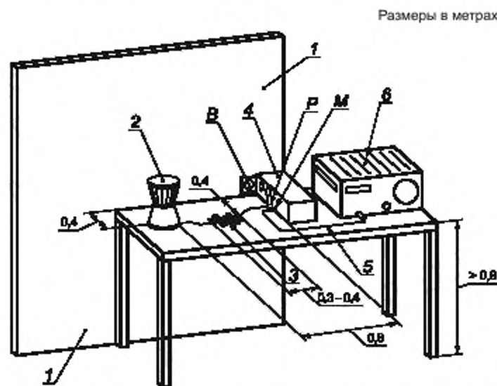
1 — металлическая стена 2 × 2 м; 2 — ИО; 3 — излишек шнура питания (например, 0,02 × 0,3 м) уложенный в форме извилины; 4 — ЗСП; 5 — коаксиальный кабель; 6 — измерительный приемник. В — соединение с опорным заземлением; М — вход измерительного приемника; Р — питание ИО. Допуски длин кабелей и расстояний должны быть такими, как это практически возможно
