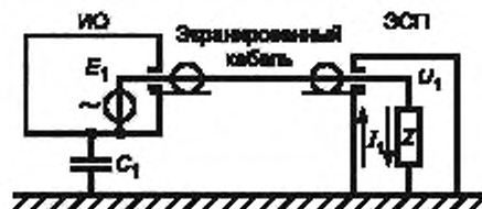
Рисунок А.1 — Общая схема хорошо экранированного ИО с недостаточной фильтрацией
