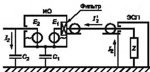
Рисунок А.4 — ИО с хорошей фильтрацией, но с неполным экранированием, с U_2 , уменьшенным до нуля
