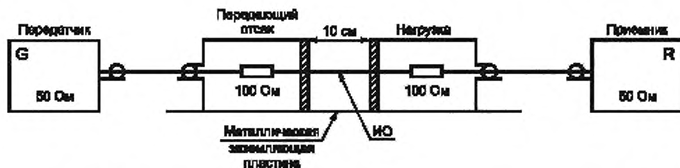
Рисунок Е.9 — Испытательная установка для измерения вносимого затухания PE-дресселей и подавителей поверхностных токов
