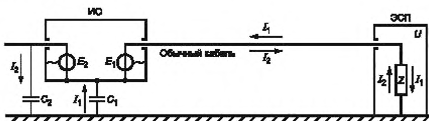
Рисунок A.7 — Поддача помехи через обычные провода
