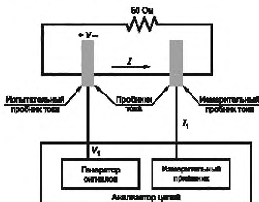
Рисунок Н.4 — Установка для калибровки
