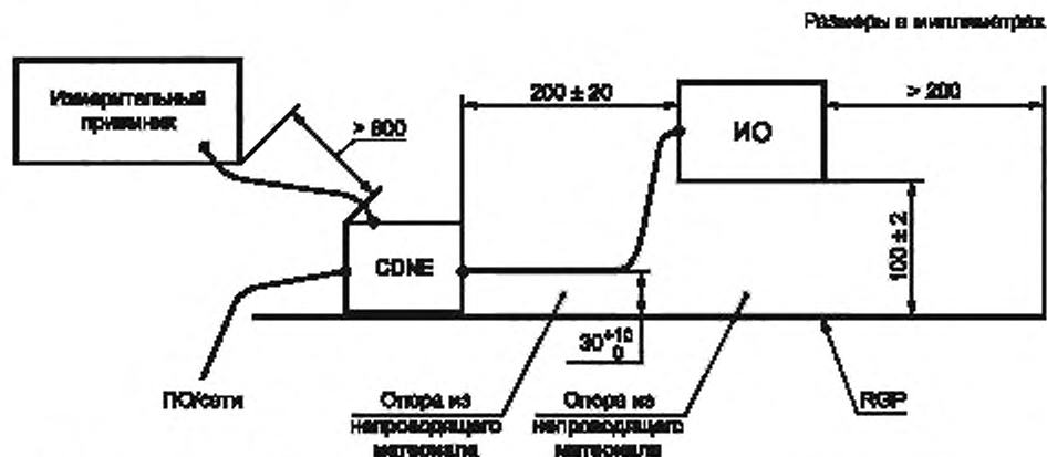
Рисунок 23 — Испытательная установка для измерений ИО с одним кабелем
