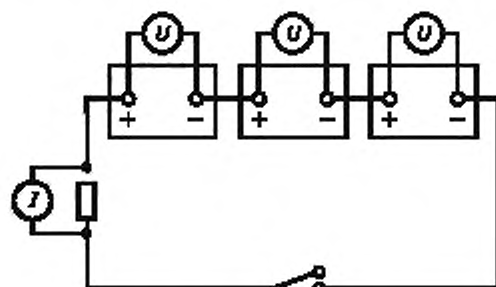
Рисунок 2 — Типичная электрическая схема при испытаниях
