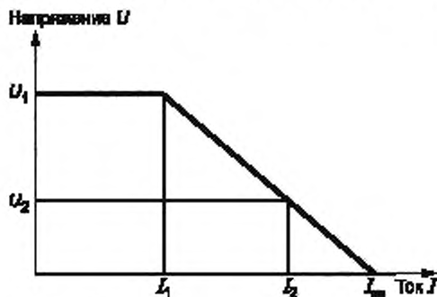
Рисунок 1 — Разрядная характеристика U = f(I)
