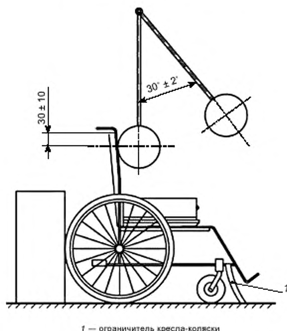
Рисунок 24 — Испытание на ударную прочность спинки кресла
