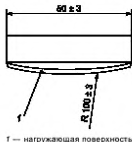
Рисунок 2 — Выпуклая нагружающая пластина
