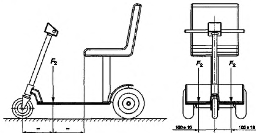
Рисунок 12 — Точки приложения испытательной нагрузки на площадку опоры-стопа скутера
