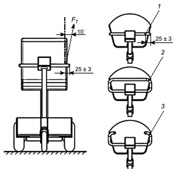
1 — точка приложения для прямых (Т) рукояток; 2 — точка приложения для рукояток, которые имеют форму петли; 3 — точка приложения для рукояток, которые имеют форму открытой петли
