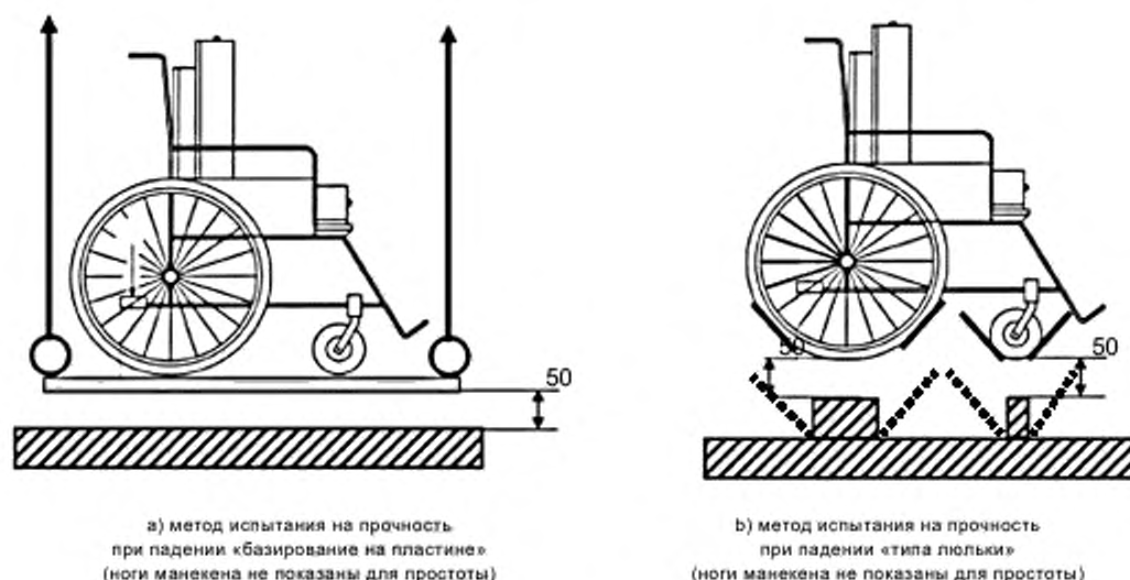
Рисунок 31 — Методы подъема колес
