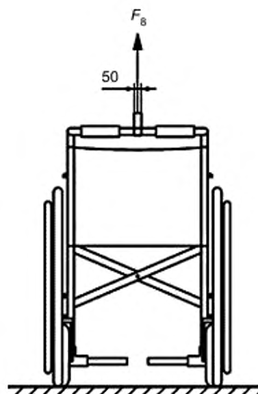
в) сила, прикладываемая к рукоятке в виде перекладки снизу вверх
