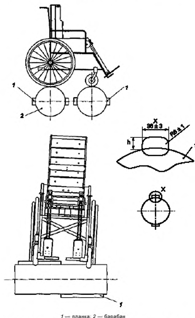
1 — планка; 2 — барабан h — 6 мм — для диаметров колес до и включая 75 мм; 9 мм — для диаметров колес более чем 75 мм, менее и включая 100 мм; 12 мм — для всех других диаметров колес более чем 100 мм. Допуск \pm 8\%
