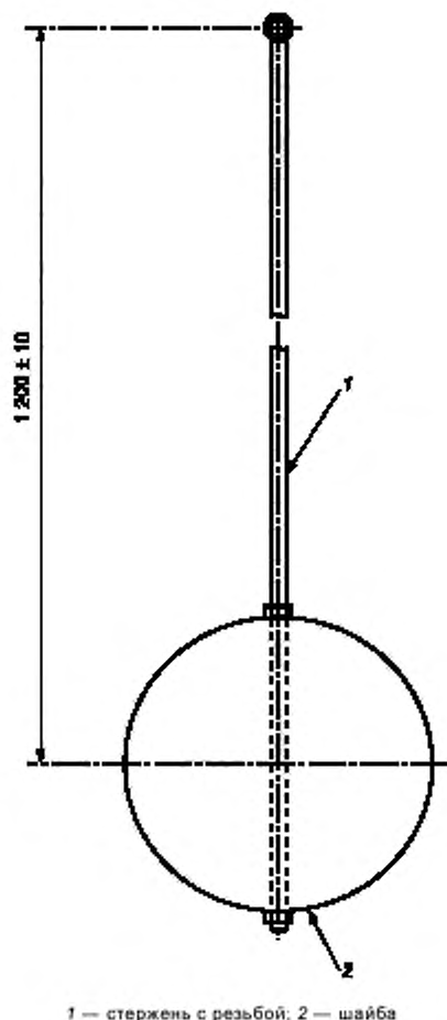
Рисунок 4 — Альтернативный маятник для испытания спинки кресла
