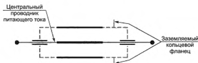
Рисунок 3 — Коаксиальный проходной конденсатор
