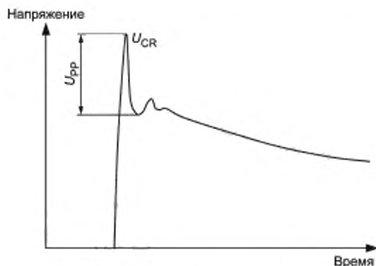
Рисунок 7 — Форма импульсной волны
