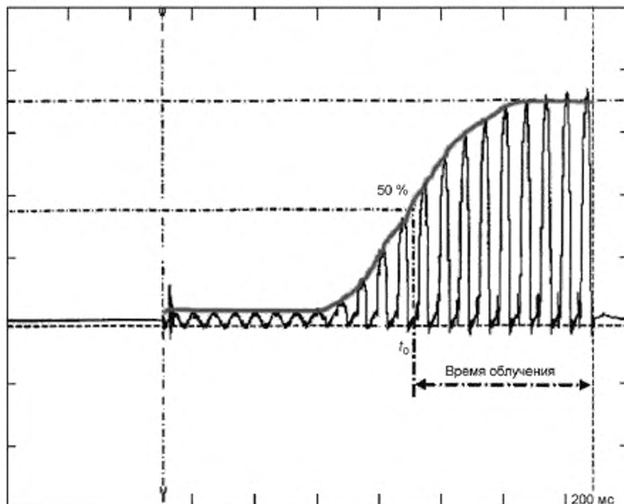
Рисунок АА.2 — ВОЗДУШНАЯ КЕРМА ПРИ ОБЛУЧЕНИИ, ПРОИЗВОДИМ ОДНОПОЛУПЕРИОДНЫМ РПУ
