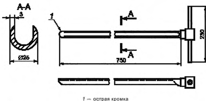
Рисунок 2 — Пробоотборник открытого типа — типичные размеры
