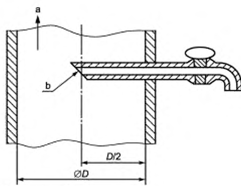
Рисунок 11 — Пробоотборник в виде крана для резервуаров или трубопроводов
