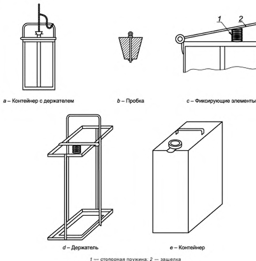
Рисунок 9 — Одноразовый контейнер-пробоотборник
