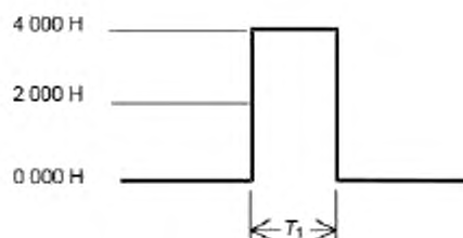
Рисунок 2 — Форма цифрового измерительного сигнала
