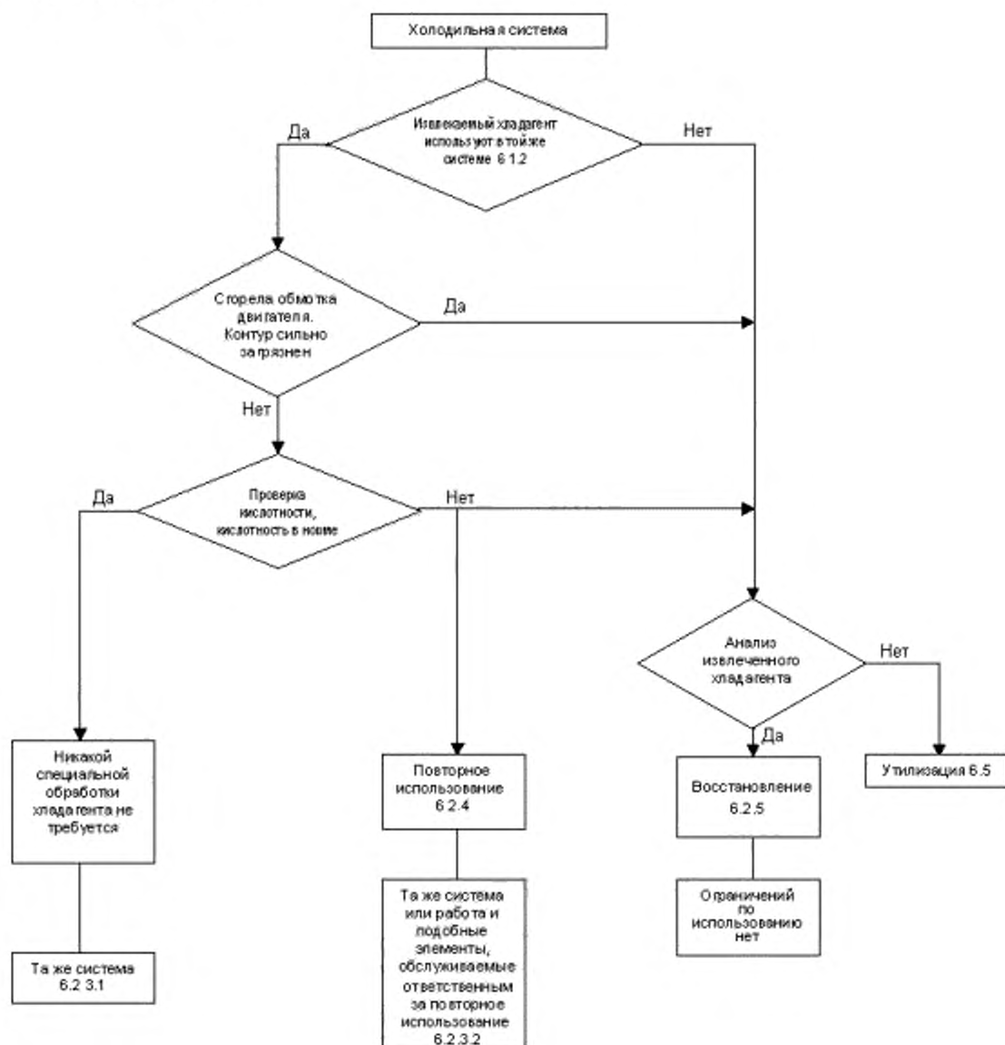
Рисунок 2 – Блок-схема операций, выполняемых при извлечении хладагента
