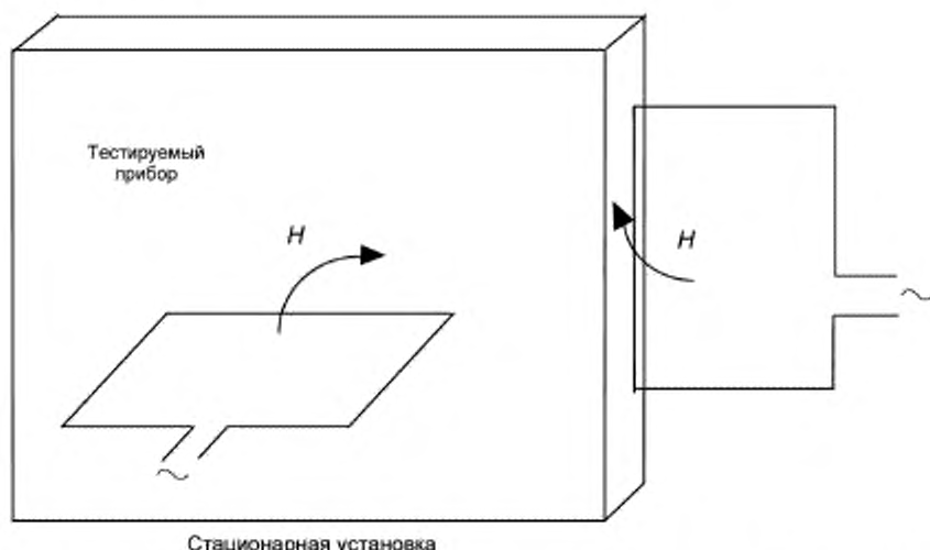
Рисунок 3б – Пример применения тестового магнитного поля с помощью метода приближения
