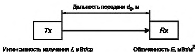
Рисунок 3 — Дальность передачи
