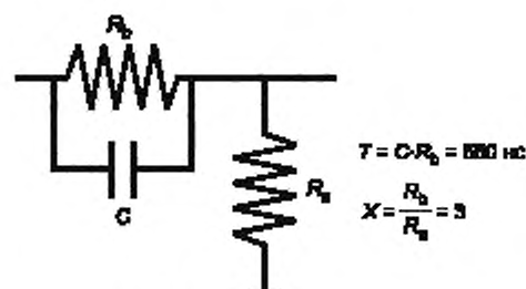
Рисунок 14 — Схема предуслаживания (пример)
