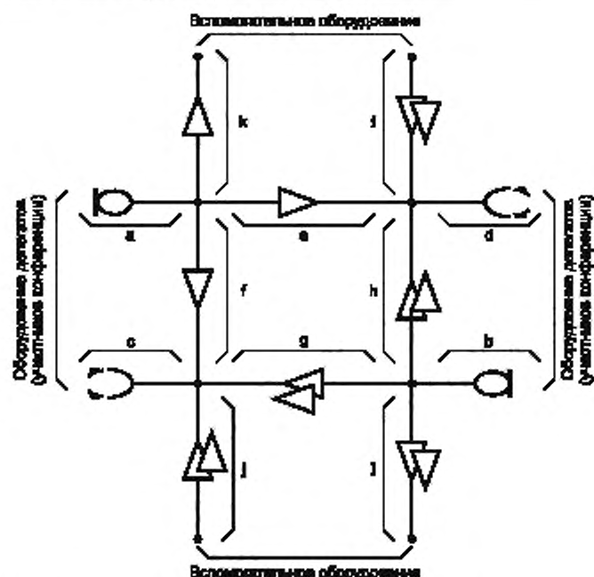
Рисунок 1 — Схемное представление звуковой системы конференц-связи
