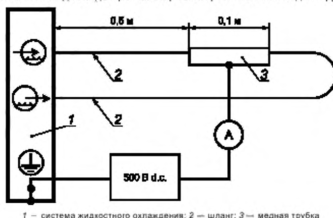
Рисунок 1 — Схема измерения тока утечки
