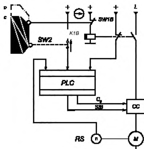
PLC — программируемый логический контроллер; CC — преобразователь тока; M — двигатель; RS — датчик вращения; o — разомкнуто; c — замкнуто; C S — функция безопасного останова (стандартная); SIB — импульс безопасной блокировки; K1B — контактор, SW1B — выключатель (нормально замкнутый); SW2 — выключатель (нормально разомкнутый)
