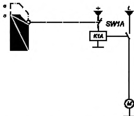
o — разомкнуто; c — замкнуто; M — двигатель; K1A — контактор; SW1A — выключатель (нормально замкнутый)
