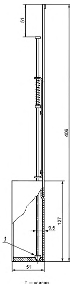
1 — клапан
