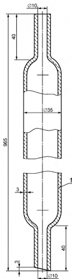
1 — стеклянная трубка, зауженная с обоих концов
