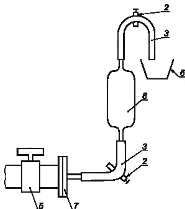
2 — запорный кран (внутренний, внешний); 3 — гибкая соединительная трубка; 5 — проботоборный кран оборудования; 6 — емкость для отходов; 7 — глухой фланец; 8 — ампула
