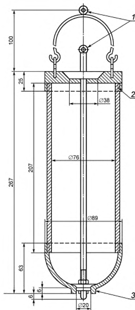
Рисунок 1 — Глубинный пробоотборник
