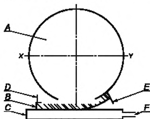
Рисунок 1 — Общий вид испытательной машины
