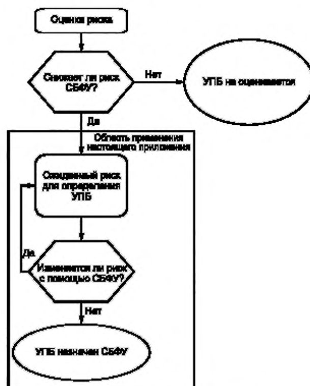
Рисунок А.1 — Структура процесса оценки УПБ
