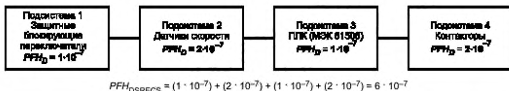
Рисунок В.8 — Оценка PFH_D для СБЭСУ
