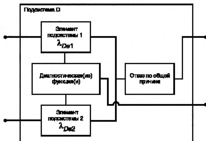
Рисунок 9 — Логическое представление подсистемы типа D
