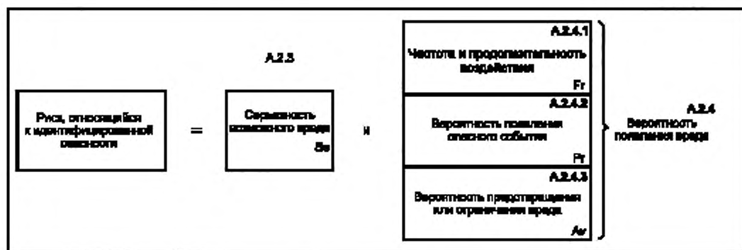
Рисунок A.2 — Параметры, используемые для оценки риска
