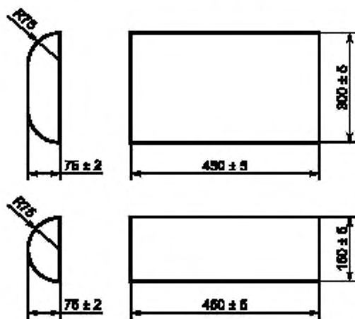
Рисунок 1 — Размеры образца
