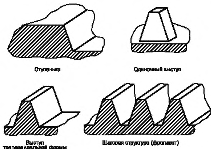
Рисунок 1 — Типовые элементы рельефа рельефной меры
