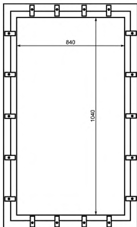
Рисунок В.2 — Наружная рама
