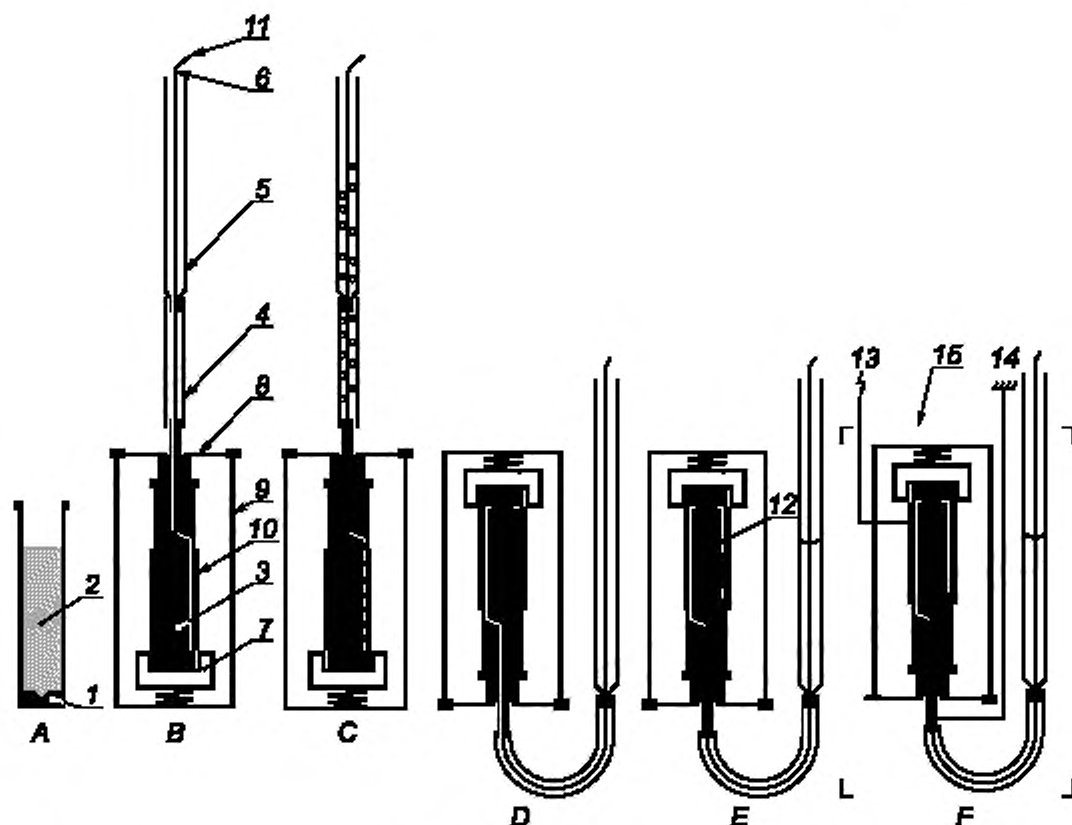
А — уровень заполнения реакционной камеры пробой масла; В — введение внутреннего электрода (с соединительным шлангом, бюреткой и капиллярной трубкой); С — насыщение испытательным газом; D — переворачивание держателя на 180° (положение при испытании); E — подача испытательного газа через капиллярную трубку; F — размещение испытательной установки в масляной бане, подача напряжения
