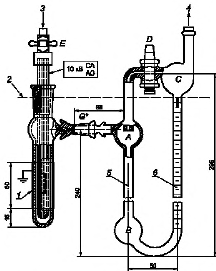
А, В, С — шарообразные расширения стеклянной трубки; D — перепускной кран; E — игольчатый вентиль; G — конусное стеклянное соединение 10/19 (по стандарту [3]); 1 — внешний электрод; 2 — уровень жидкости в масляной бане; 3 — подача газа; 4 — в атмосферу; 5, 6 — прозрачная трубка внутренним диаметром 5 мм и наружным диаметром 7 мм по стандарту [1]
