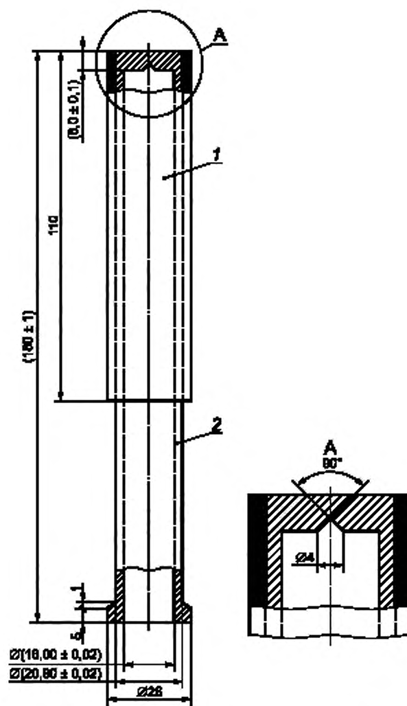
Рисунок 4 — Реакционная камера
