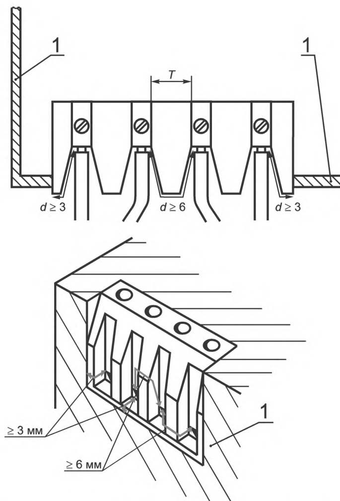
1 — токопроводящая часть; T — электрические зазоры и длины путей утечки в соответствии с 6.3; d — электрические зазоры на внешних соединительных устройствах зажимов в соответствии с 6.2.1.
