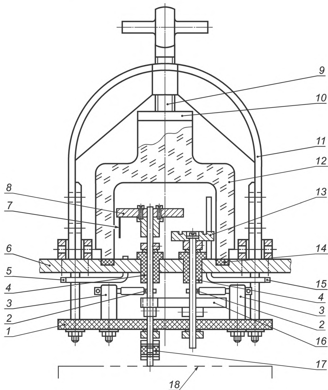
1 — изолирующая пластина; 2 — подвод тока; 3 — изолированный болт; 4 — изолированный подшипник; 5 — выходное отверстие для газа; 6 — цоколь основания; 7 — вольфрамовая проволочка; 8 — держатель проволочек; 9 — зажимной винт; 10 — нажимная пластина; 11 — зажим; 12 — камера; 13 — кадмиевый контактный диск; 14 — резиновое уплотнение; 15 — входное отверстие для газа; 16 — шестерня с соотношением зубьев 50:12 м; 17 — изолированная муфта; 18 — приводной двигатель с редуктором 80 об/мин
