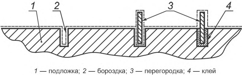
Рисунок С.3 — Измерение длины путей утечки
