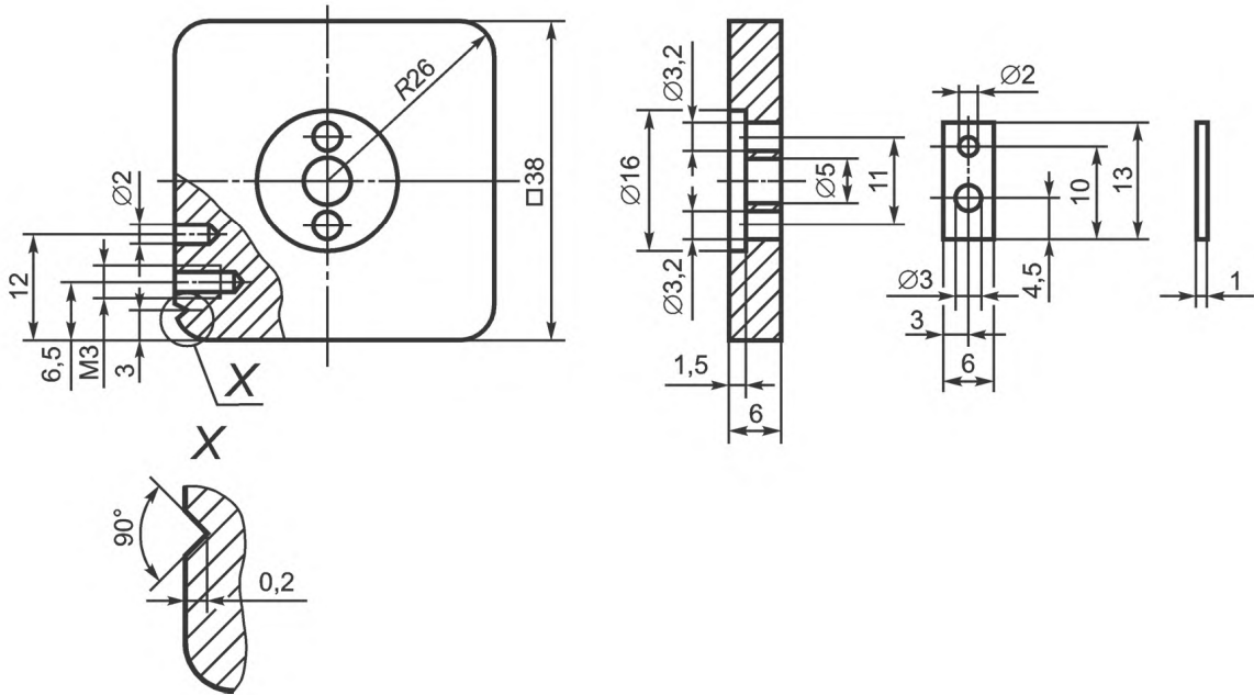
Рисунок В.3 — Держатель проволочек
