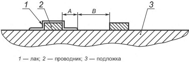
Рисунок С.4 — Измерение сложных расстояний
