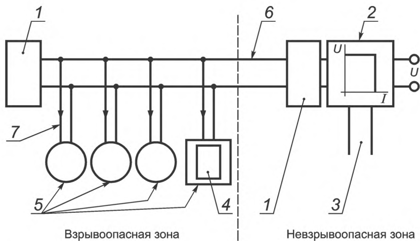
1 — оконечное согласующее устройство; 2 — источник питания; 3 — данные; 4 — переносное оконечное согласующее устройство; 5 — полевые устройства; 6 — магистральный кабель; 7 — ответвительный кабель
