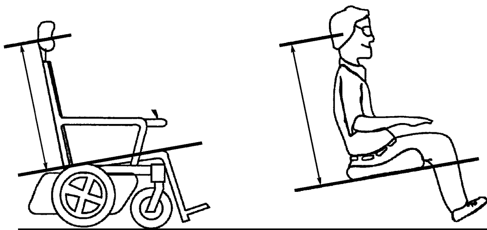
Рисунок 18 — Высота подголовника
