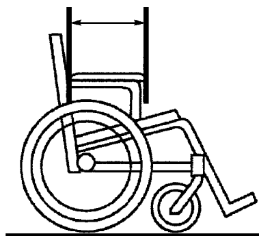
Рисунок 15 — Длина подлокотника
