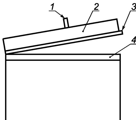
1 — рапель; 2 — трафаретная рама; 3 — устройство автоматического отключения; 4 — печатный стол
