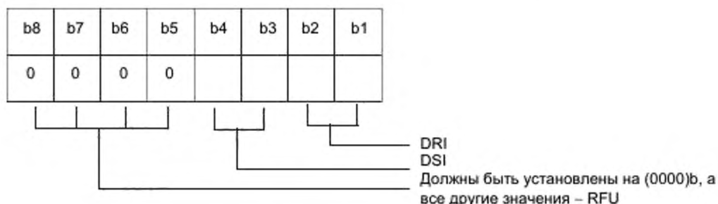
Рисунок 12 – Кодирование PPS1
