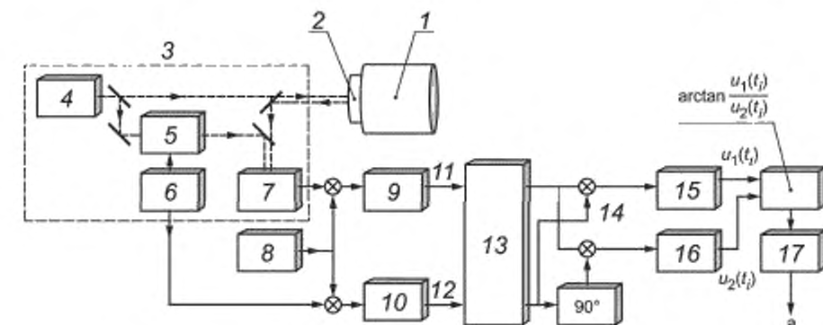
1 — вибростенд; 2 — отражатель; 3 — интерферометр; 4 — лазер; 5 — оптоакустическая ячейка Брэгга; 6 — кварцевый генератор; 7 — фотодетектор; 8 — синтезирующий генератор; 9 — фильтр нижних частот; 10 — фильтр нижних частот; 11 — измерительный сигнал; 12 — опорный сигнал; 13 — устройство регистрации; 14 — синтез квадратурных сигналов; 15 — фильтр нижних частот; 16 — фильтр нижних частот; 17 — устройство обработки (преобразования); а — результат измерения (параметр вибрации или удара)
