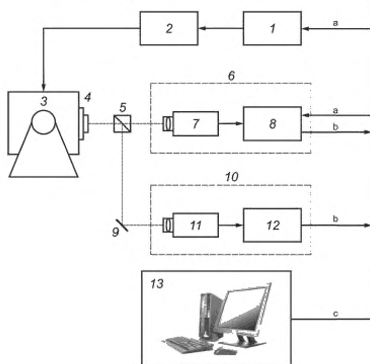
1 – генератор сигналов; 2 – усилитель мощности; 3 – вибростенд; 4 – стол с отражателем; 5 – светоделитель; 6 – ЗЛВ; 7 – оптический преобразователь; 8 – сигнальный процессор; 9 – регулируемое зеркало; 10 – калибруемый лазерный виброметр; 11 – оптический преобразователь; 12 – сигнальный процессор; 13 – система управления и сбора данных; а – шина управления; б – сигнальная шина, с – цифровой интерфейс
