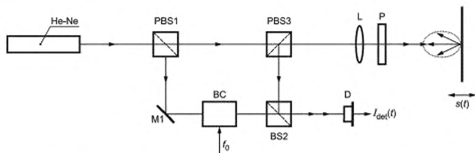
BC — акустооптическая ячейка Брэгга; BS — светоделитель; D — детектор; He-Ne — лазер; L — линза; M — зеркало. P — четвертьволновая пластина, PBS — поляризационный светоделитель
