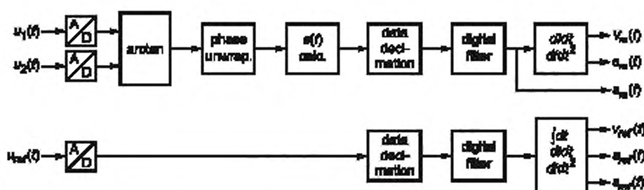
a_m(t) — измеряемое ускорение; a_{ref}(t) — опорное ускорение; s_m(t) — измеряемое перемещение; s_{ref}(t) — опорное перемещение; t — время; u_1, u_2 — два квадратурных сигнала, u_{ref}(t) — сигнал опорного напряжения; v_m(t) — измеряемая скорость; v_{ref}(t) — опорная скорость
