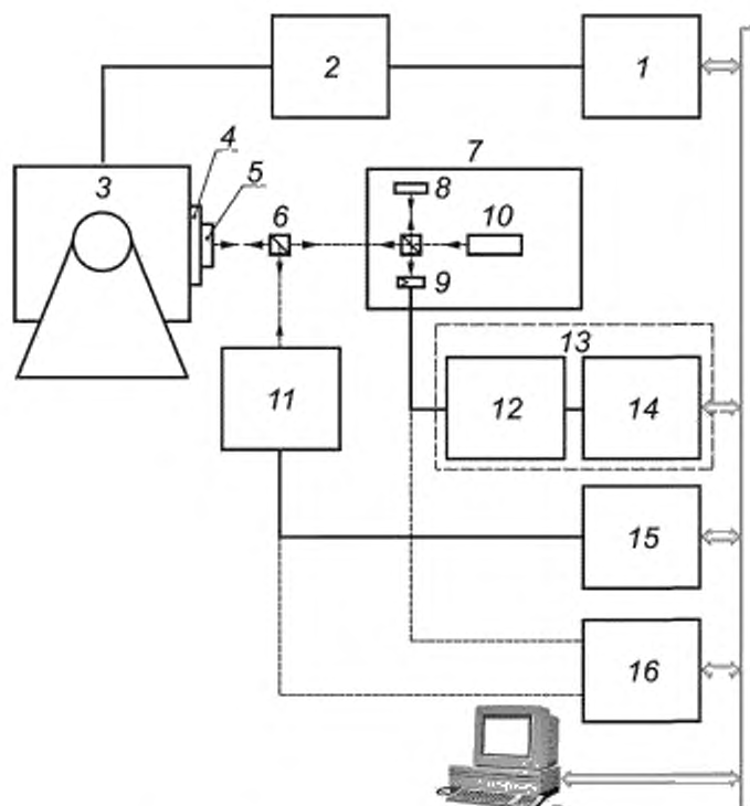
1 — генератор сигналов, 2 — усилитель мощности, 3 — вибростенд; 4 — стол вибростенда; 5 — отражатель; 6 — светодетектор, 7 — интерферометр; 8 — опорное зеркало. 9 — фотодетектор; 10 — лазер; 11 — калибруемый лазерный виброметр; 12 — полосовой фильтр, настроенный на частоту вибрации; 13 — анализатор частоты, 14 — вольтметр, 15 — вольтметр 16 — осциллограф
