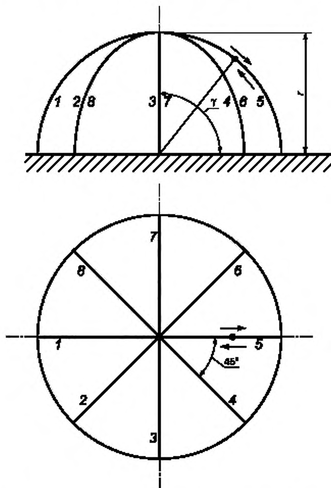
Рисунок G.1 — Меридиональные траектории на полусфере
