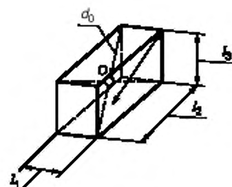
а) Заглушенная камера, d_0 = \sqrt{(l_1/2)^2 + (l_2/2)^2 + (l_3/2)^2}
