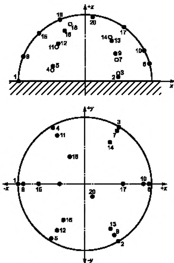
Рисунок E.2 — Точки измерений на полусферической измерительной поверхности (случай источника широкополосного шума)
