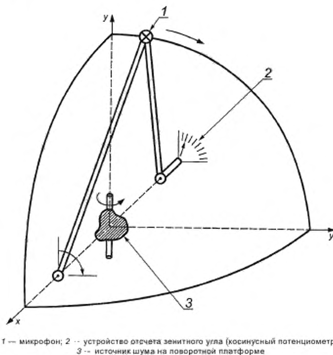
Рисунок G.2 — Пример механической системы перемещения микрофона по меридиональной траектории
