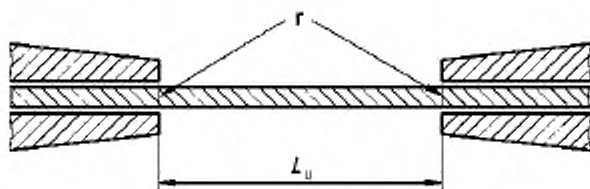
r — ограничительные отметки для стандартного испытания; L_u — эффективная длина, измеренная без нагрузки
