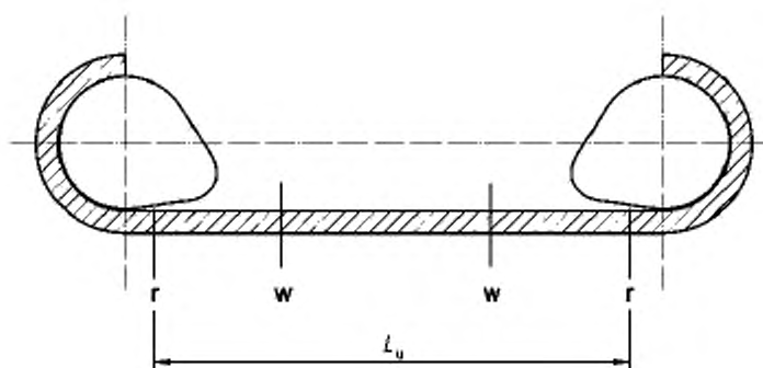
r — ограничительные отметки для стандартного испытания; L_u — эффективная длина, измеренная без нагрузки; w — ограничительные отметки для l_0
