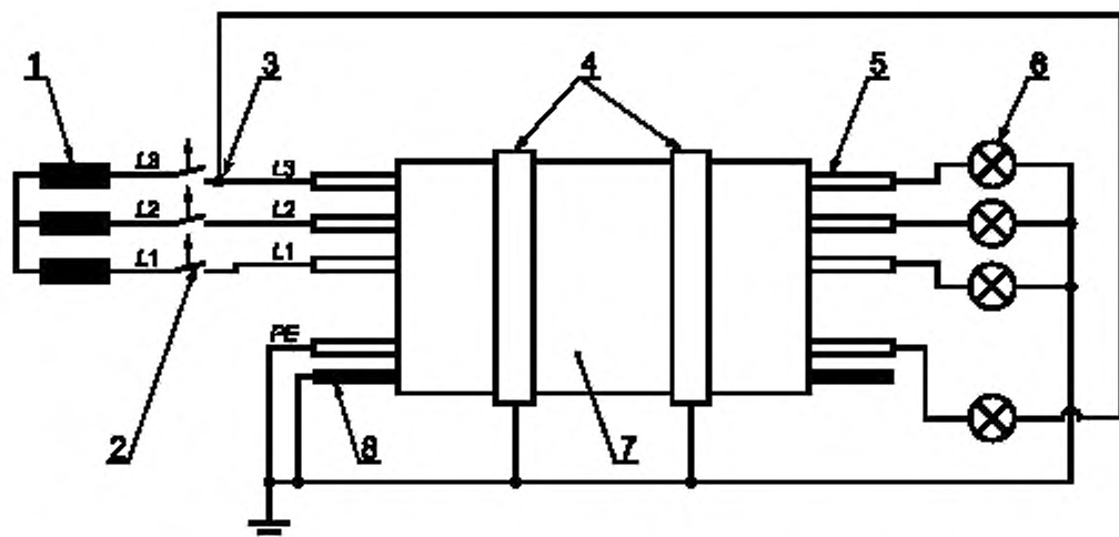
1 — трансформатор; 2 — плавкий предохранитель (2 А); 3 — подключение к линии L3 (или L1, или L2); 4 — поддерживающие кольца; 5 — испытываемая жила или группа жил; 6 — нагрузочный индикаторный прибор (например, лампа); 7 — образец; 8 — металлический экран (если имеется); L1, L2, L3 — линии испытываемых жил или групп жил (L2, L3, если имеются); PE — жила заземления (если имеется)
