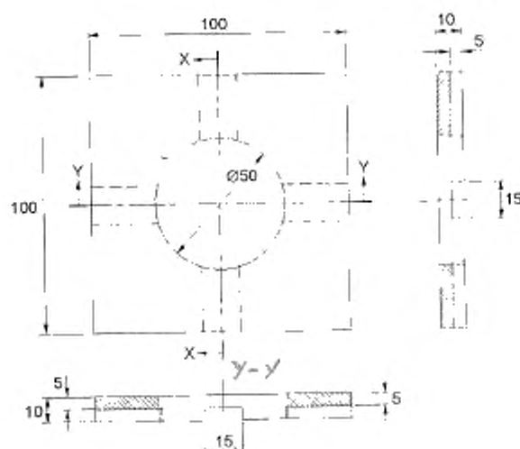
Рисунок 113а – Фрагмент А – Нижняя часть маски
