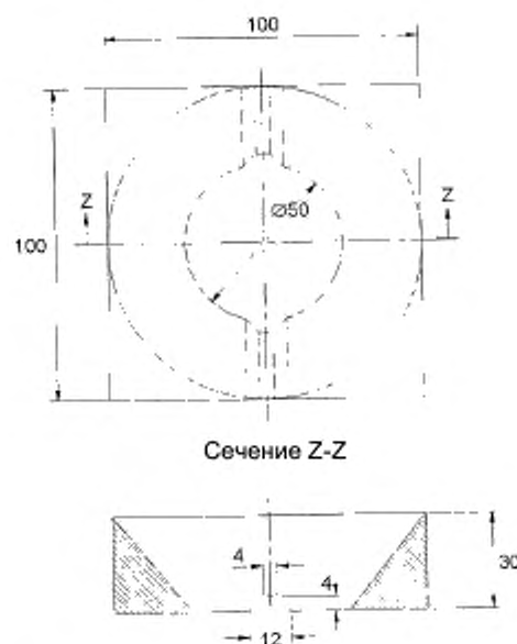
Рисунок 113б – Фрагмент В – Верхняя часть маски
