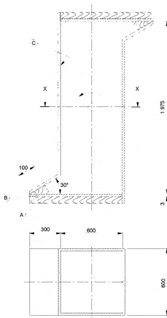
Рисунок 107 – Вращающийся барабан для испытания механической прочности подушек
