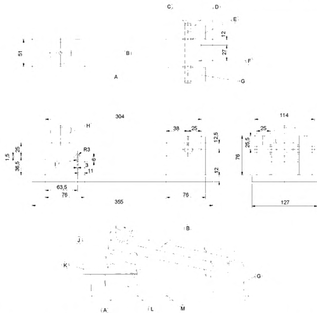
А – основание; В – рычаг; С – неплотно пригнанный штифт; D – утопленное смазочное отверстие; E – механически обработанная шайба; F – отверстие с внутренней резьбой для установочных винтов; G – опора рычага; H – ручка; I – паз; J – образец; K – картон; L – опора; M – скобы
