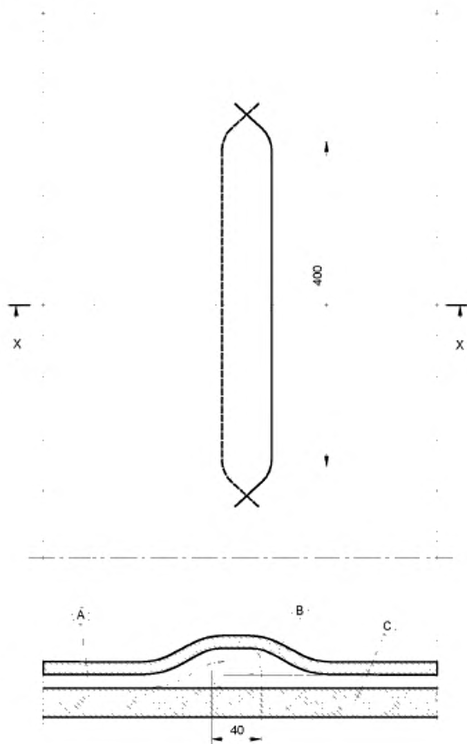
Рисунок 104 – Подготовка к испытаниям с тройным изгибом
