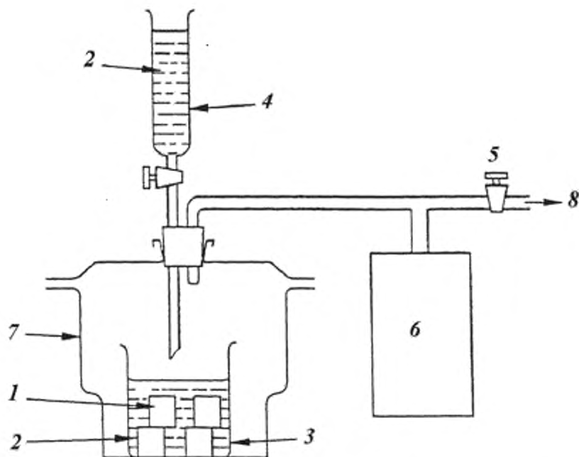
1 – испытуемый образец; 2 – насыщающая жидкость; 3 – стакан; 4 – разделительная воронка; 5 – запорный клапан вакуумного насоса; 6 – устройство измерения давления (например, манометр); 7 – эксикатор; 8 – удаление воздуха (к вакуумному насосу)
