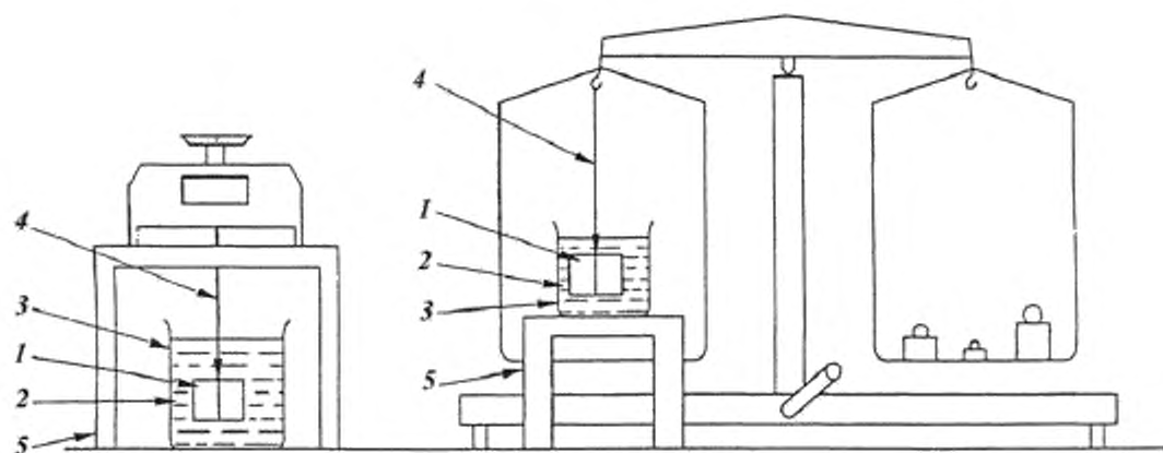
1 – испытуемый образец; 2 – насыщающая жидкость; 3 – стакан; 4 – подвесная нить; 5 – подставка
