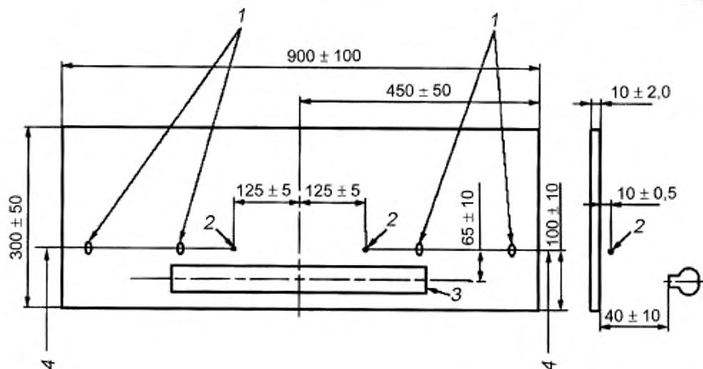
1 — опоры для термопар; 2 — кончик термопары; 3 — горелка; 4 — термопара типа К диаметром 1,5 мм в оболочке
