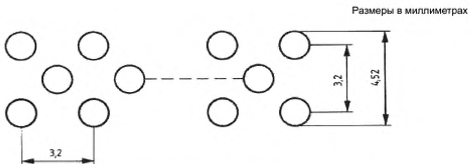
Рисунок 5 — Фронтальная поверхность рабочей части горелки
