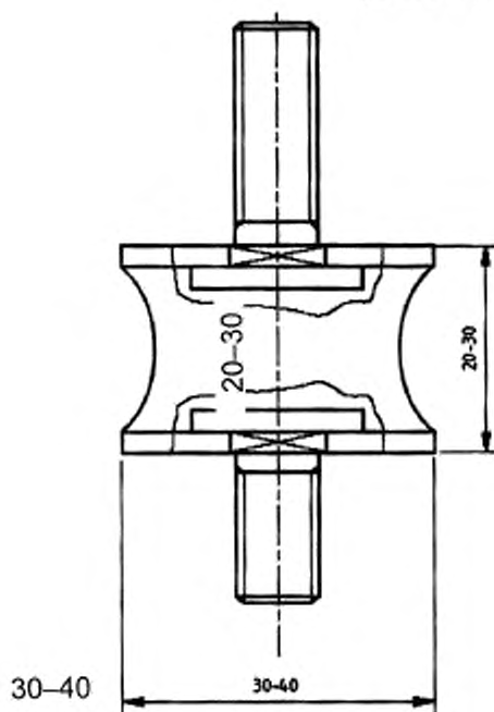
Рисунок 4 — Типичная резиновая втулка для крепления испытательной панели
