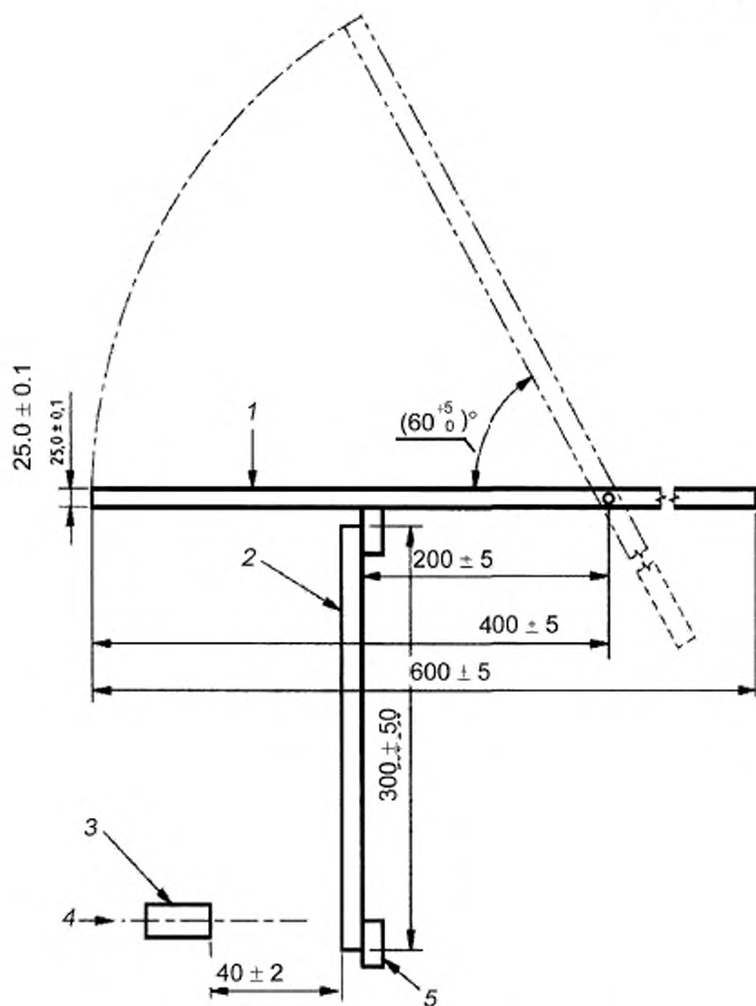
1 — ударное устройство; 2 — панель; 3 — газовая горелка; 4 — осяевая линия фронтальной поверхности горелки; 5 — жесткая опора
