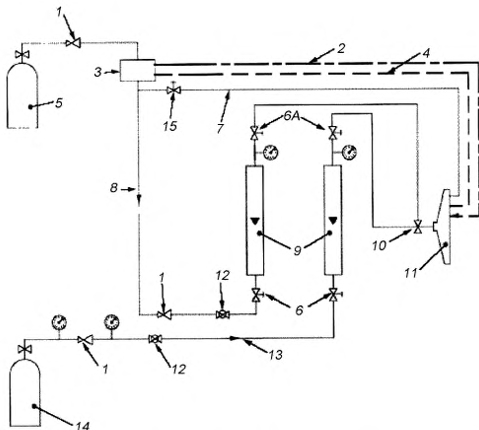
1 — редуктор; 2 — пьезоэлектрический воспламенитель; 3 — устройство для прерывания работы горелки; 4 — контрольные термопары; 5 — баллон с пропаном; 6 — винтовой клапан (6А — альтернативное расположение); 7 — вспомогательное питание; 8 — поступление газа; 9 — расходомер типа ротаметр; 10 — смеситель Вентури; 11 — горелка; 12 — шаровый вентиль; 13 — система подачи воздуха; 14 — баллон со сжатым воздухом; 15 — винтовой клапан предпускового питания
