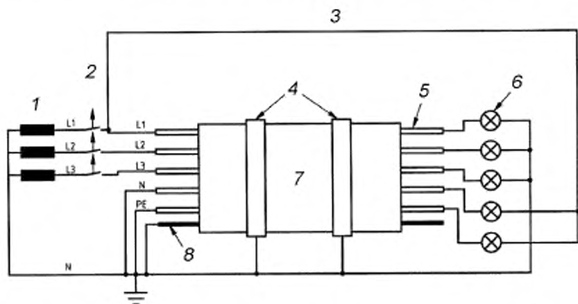
1 — трансформатор; 2 — плавкий предохранитель (2 А); 3 — фазы L1, L2 или L3; 4 — металлические зажимы; 5 — испытываемая жила или группа жил; 6 — нагрузочный индикаторный прибор; 7 — образец; 8 — металлический экран (при наличии); L1, L2, L3 — фазные жилы (L2, L3 при наличии); N — нейтральная жила (при наличии); PE — защитная жила (при наличии)
