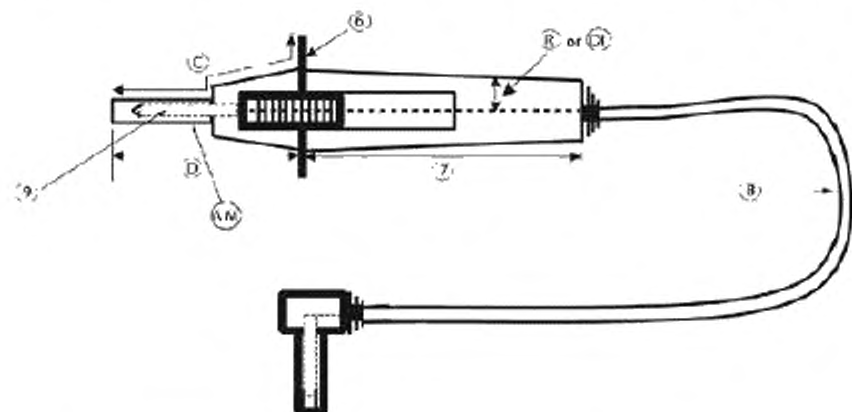
Рисунок 1б – Иллюстрация электрической изоляции пробника с отсоединяемым проводом
