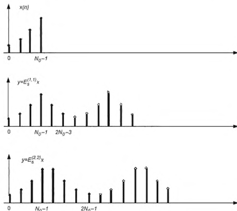
Рисунок Е.3 — Симметричное ДВП расширение
