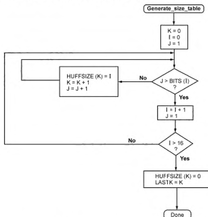
Рисунок Е.18 — Создание таблицы размеров кодов Хаффмана
