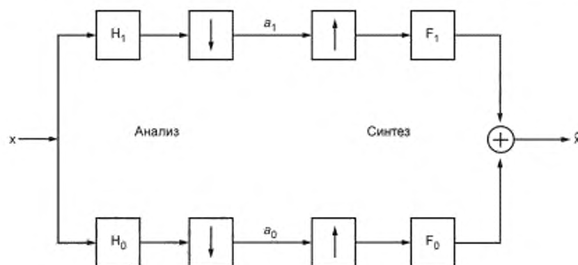
Рисунок Е.2 — Двухканальный многополосный кодер
