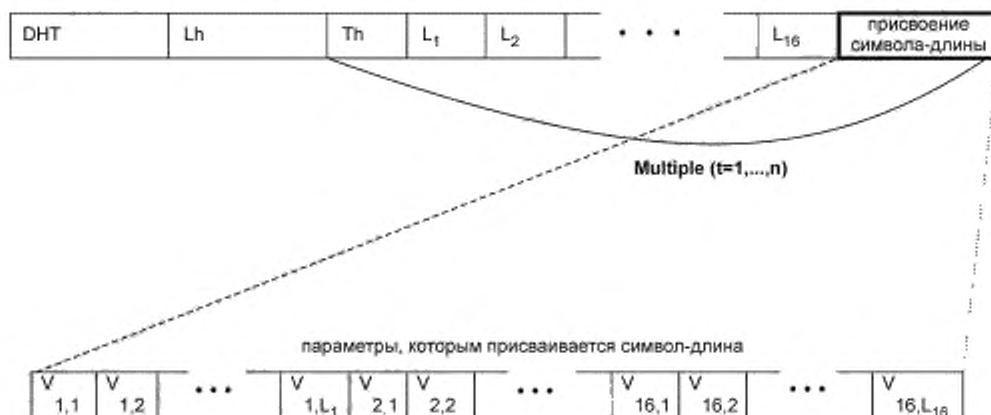
Рисунок Е.14 — Синтаксическая структура спецификации таблицы Хаффмана
