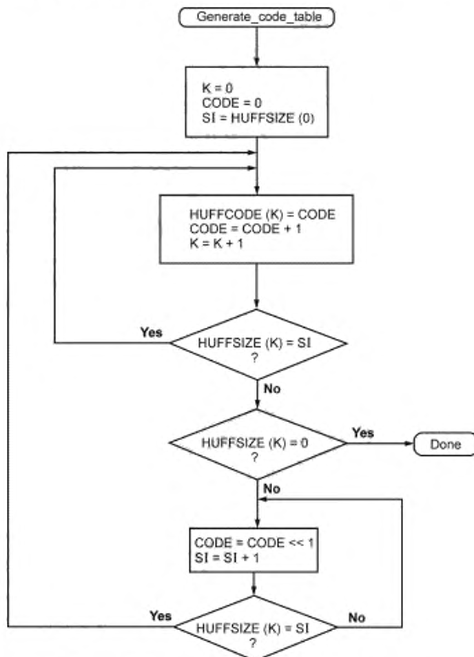
Рисунок E.19 — Создание таблицы кодов Хаффмана
