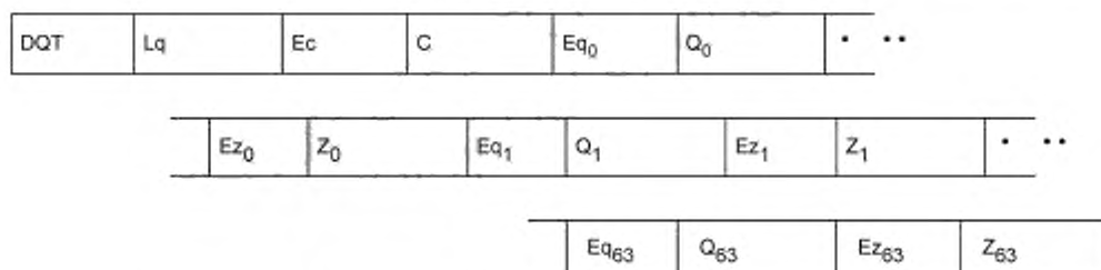
Рисунок Е.13 — Синтаксическая структура спецификации таблицы квантования
