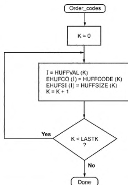
Рисунок Е.20 — Процедура упорядочения для таблиц кодов процедуры кодирования
