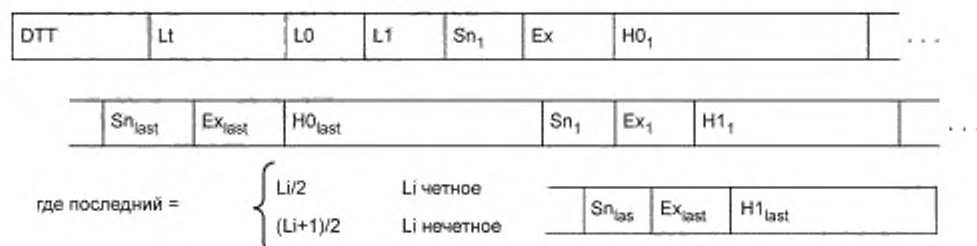
Рисунок Е.12 — Синтаксическая структура таблицы преобразования
